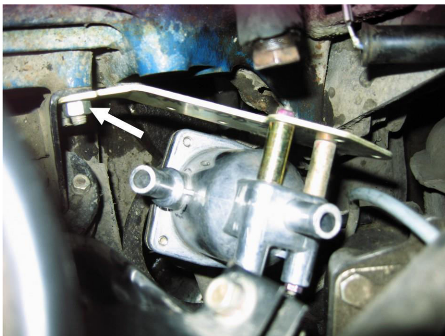
Рисунок 2. Установка подогревателя.
