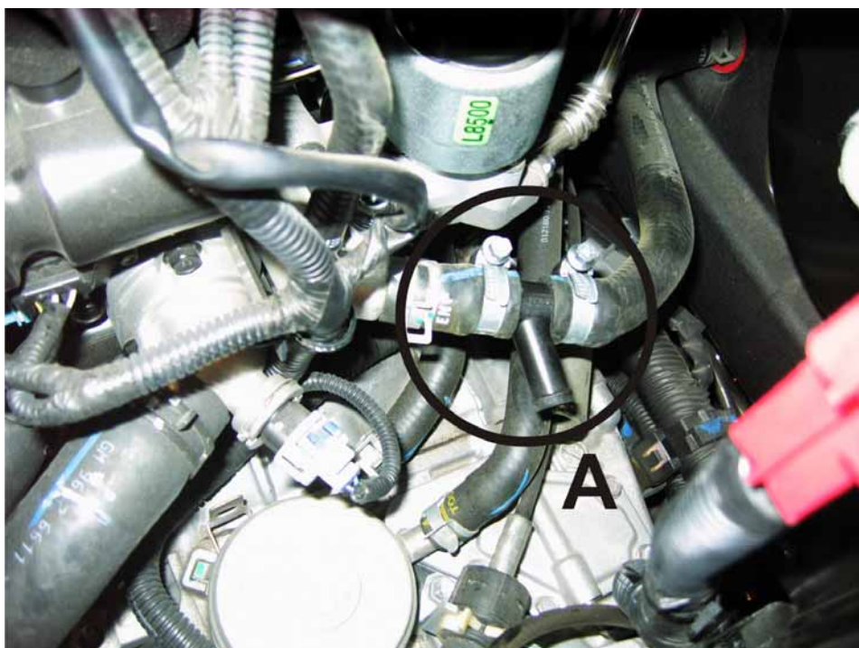
Рисунок 3. Врезка тройника выходного рукава.
