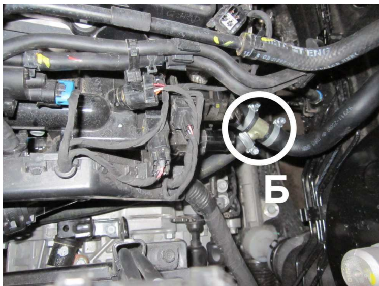
Рисунок 3. Врезка входного рукава. Вид сверху стороны аккумулятора.
