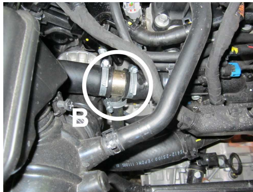
Рисунок 4. Врезка выходного рукава Вид сверху со стороны аккумулятора
