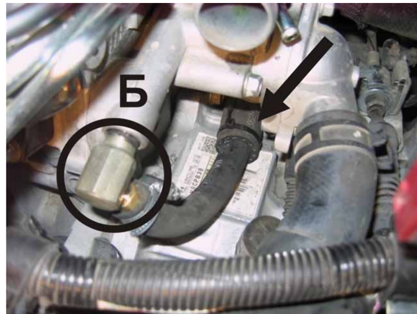
Рисунок 5. Врезка выходной магистрали. Вид снизу. Верхний шланг радиатора снят.
