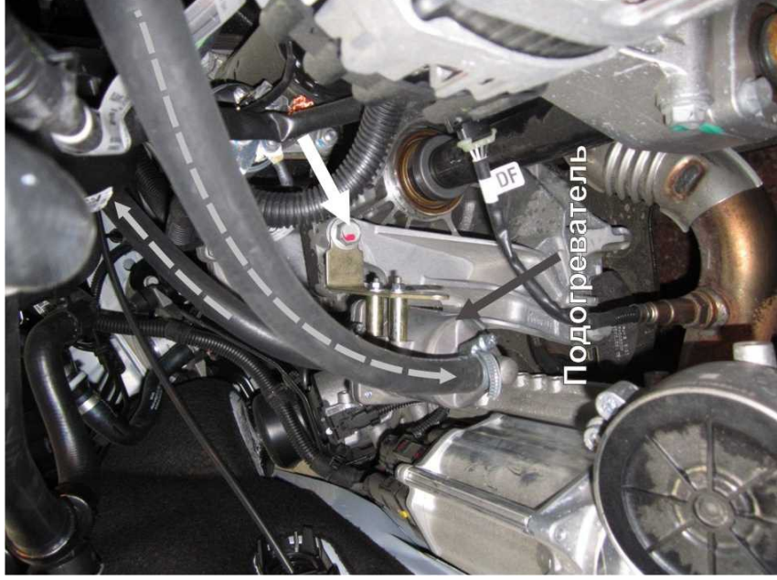
Рис. 3. Установка подогревателя на двигатель и салон автомобиля. Вид сверху со стороны правого двигателя. Установка подогревателя на
