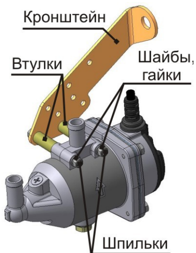
Рисунок 1. Крепление кронштейна.
