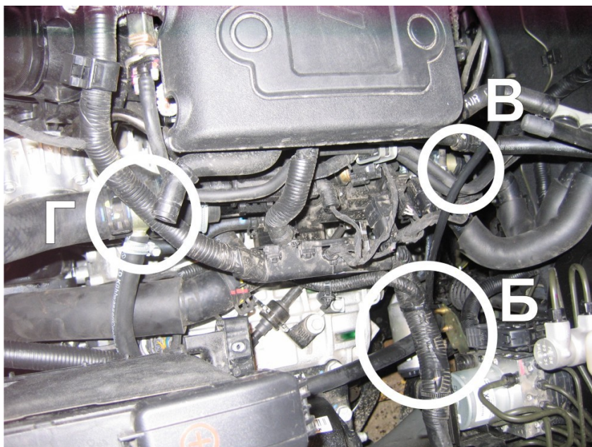
Рисунок 5. Общая картина. Вид сверху слева.
