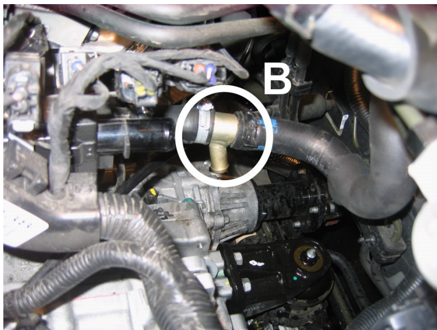
Рисунок 3. Врезка тройника входного рукава. Вид сверху слева.
