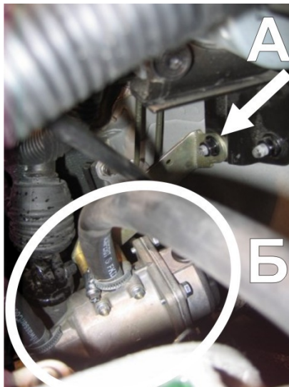
Рисунок 2. Установка подогревателя.
