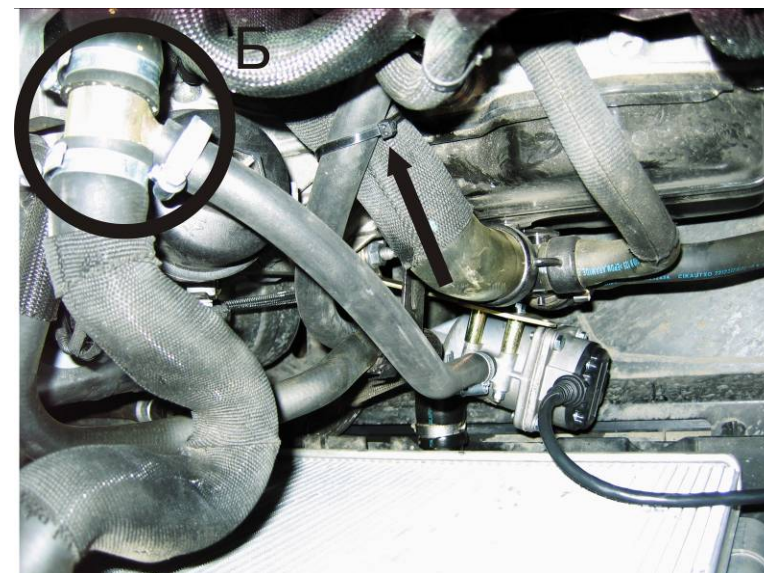
Рисунок 4. Врезка тройника выходного рукава
