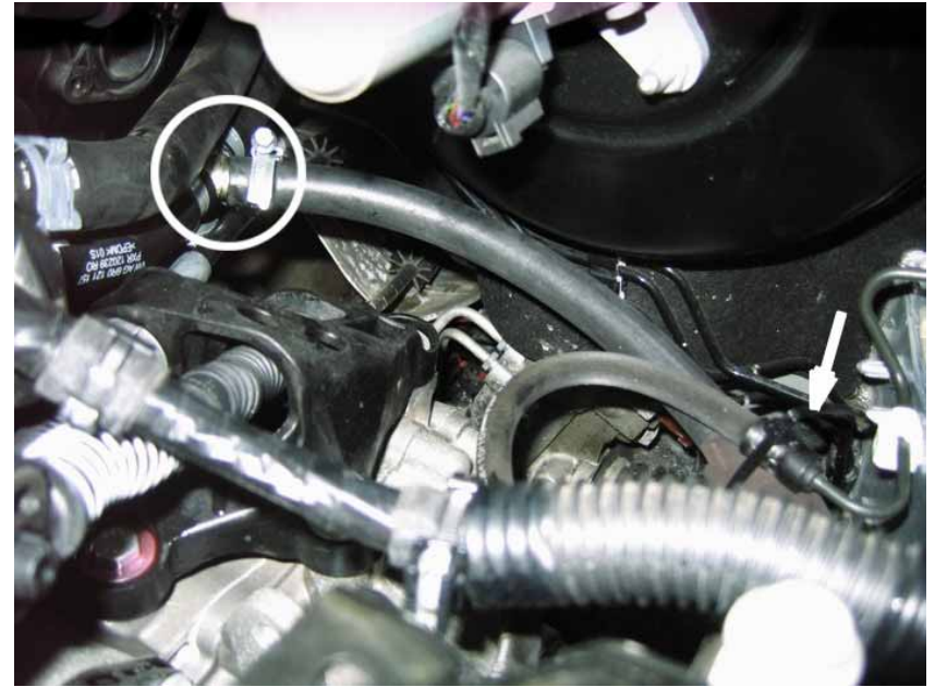
Рисунок 3. Вид сверху.
