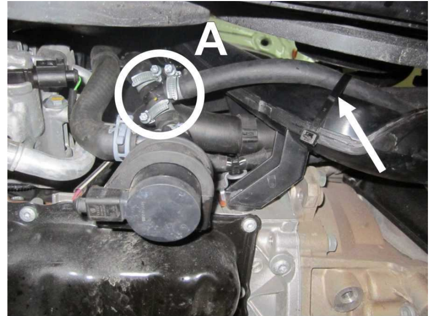
Рисунок 3. Установка тройника входного рукава. Вид снизу.
