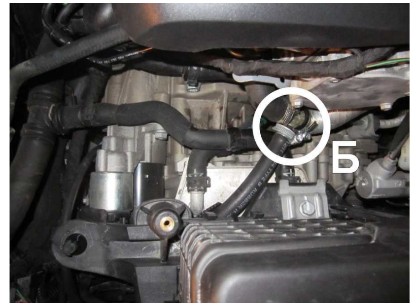
Рисунок 4. Установка тройника выходного рукава. Вид сверху со стороны аккумулятора.
