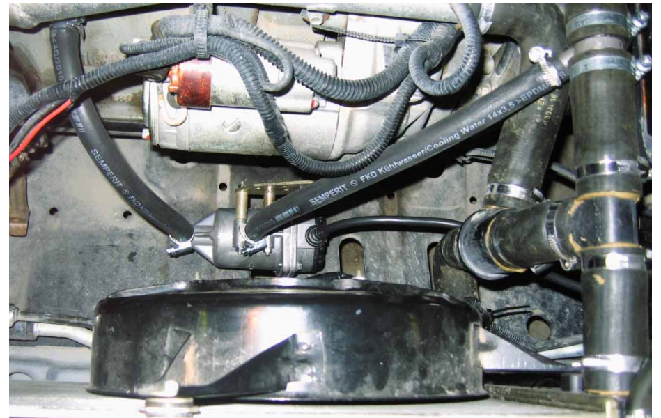
Рисунок 4 Общая сборка
