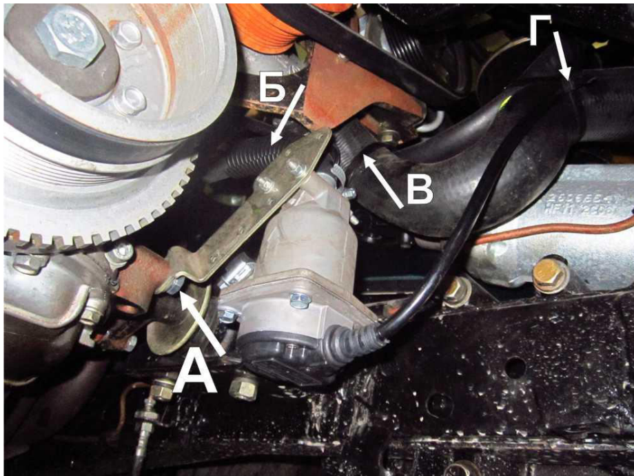
Рисунок 2. Установка подогревателя на автомобиль. Вид снизу.
