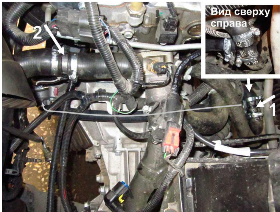
Рис. 3. Лада Калина. Врезка тройников. (Вид сверху).
